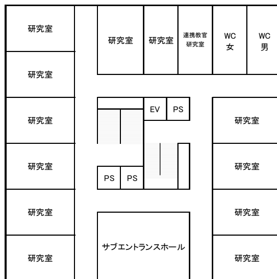
3F
